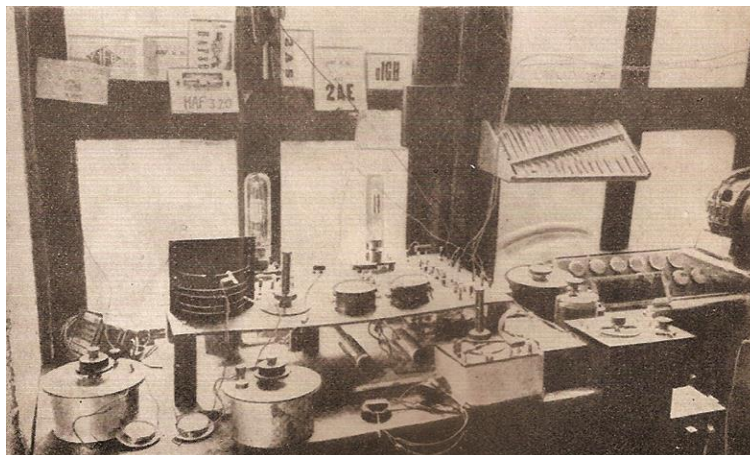
Primul post de radio-emisie pe unde scurte construit la Institutul Electrotehnic
